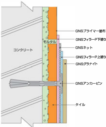
施工断面図
